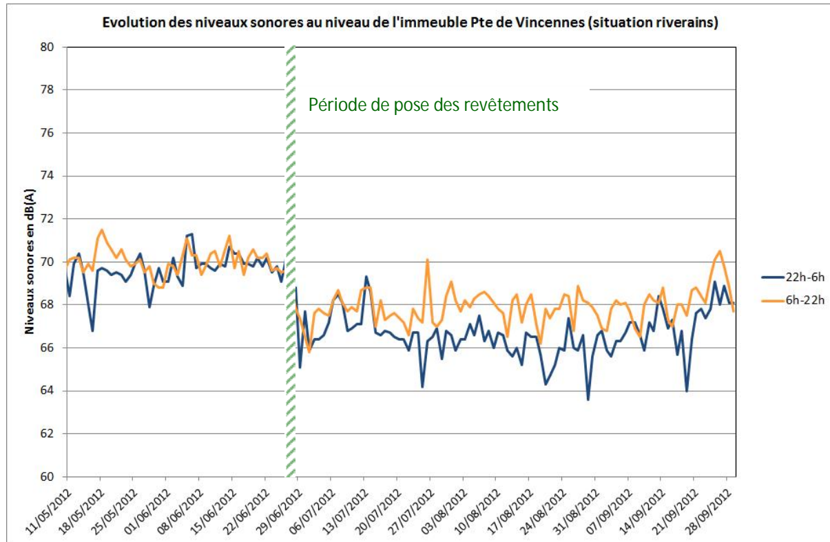
Figure 53 : Niveaux de bruit diurnes et nocturnes avant et après la pose des revêtements au niveau de la station de mesure située en façade de l'immeuble Porte de Vincennes.
