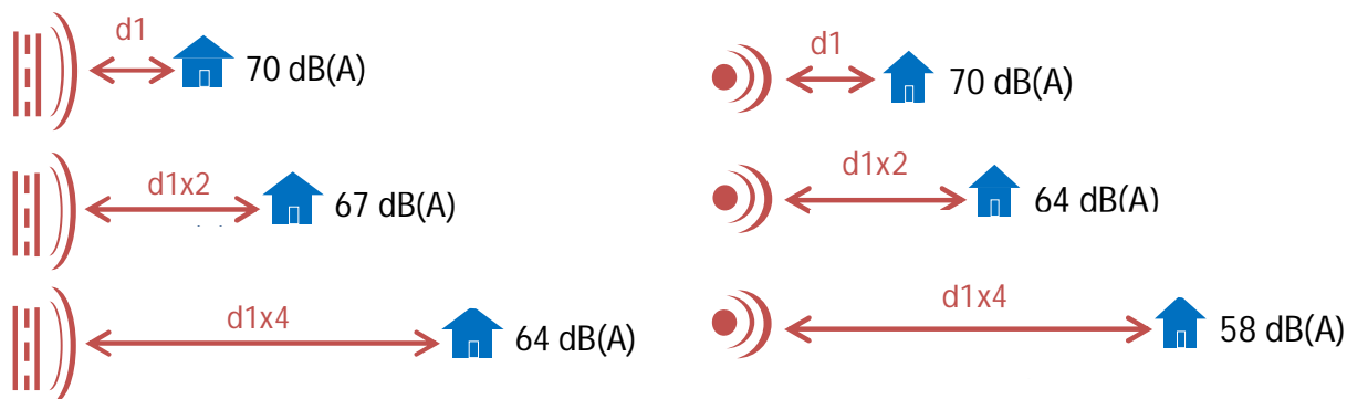
Figure 6 : Décroissance du bruit en fonction de la distance (cas d'une source linéique à gauche, cas d'une source ponctuelle à droite).
