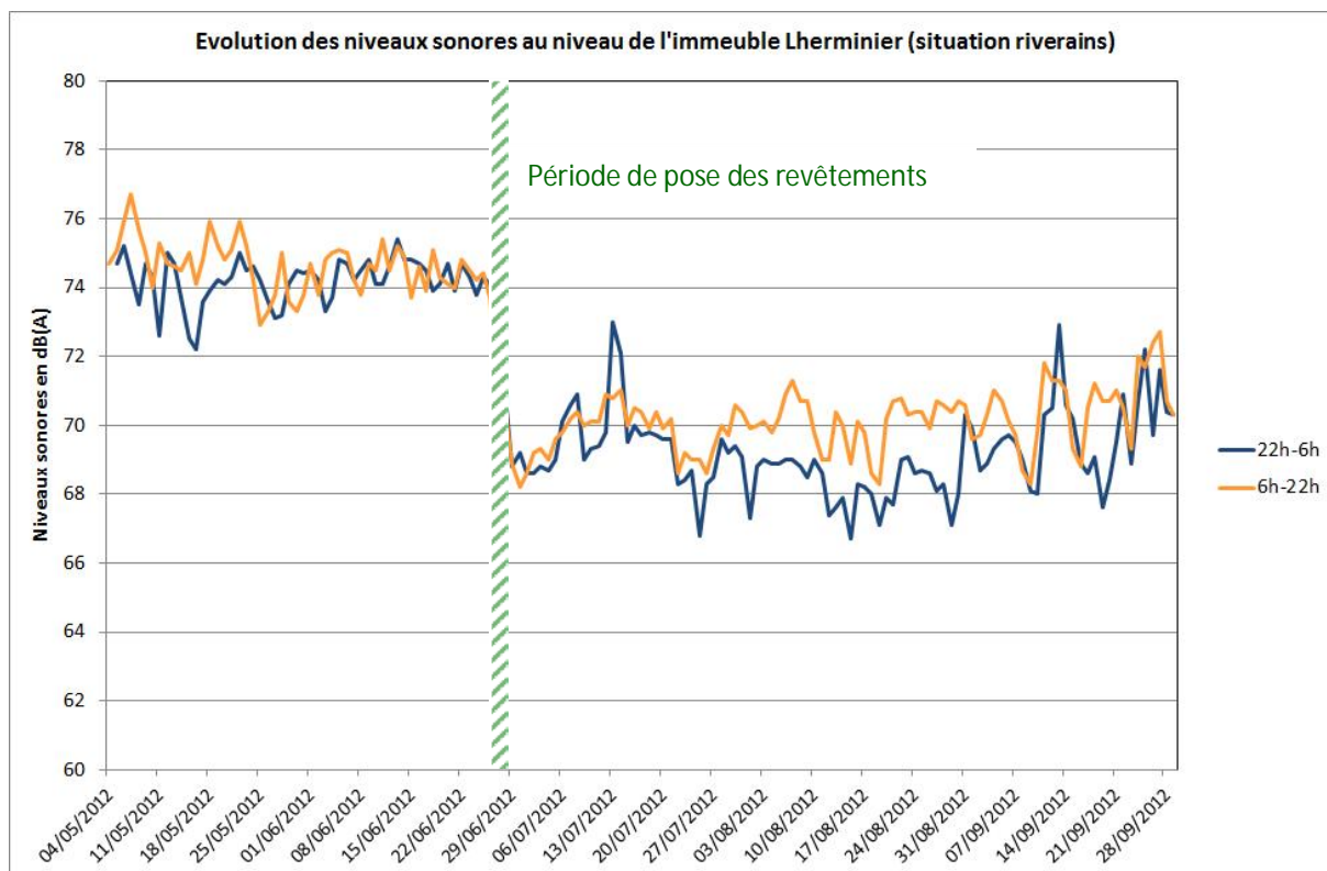
Figure 52 : Niveaux de bruit diurnes et nocturnes avant et après la pose des revêtements au niveau de la station de mesure située en façade de l'immeuble l'Herminier.
