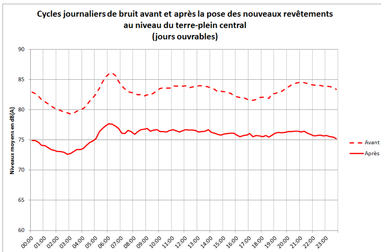
Figure 42 : Variation des niveaux au cours d'un jour ouvrable type avant et après la pose des revêtements en situation de proximité au trafic.
