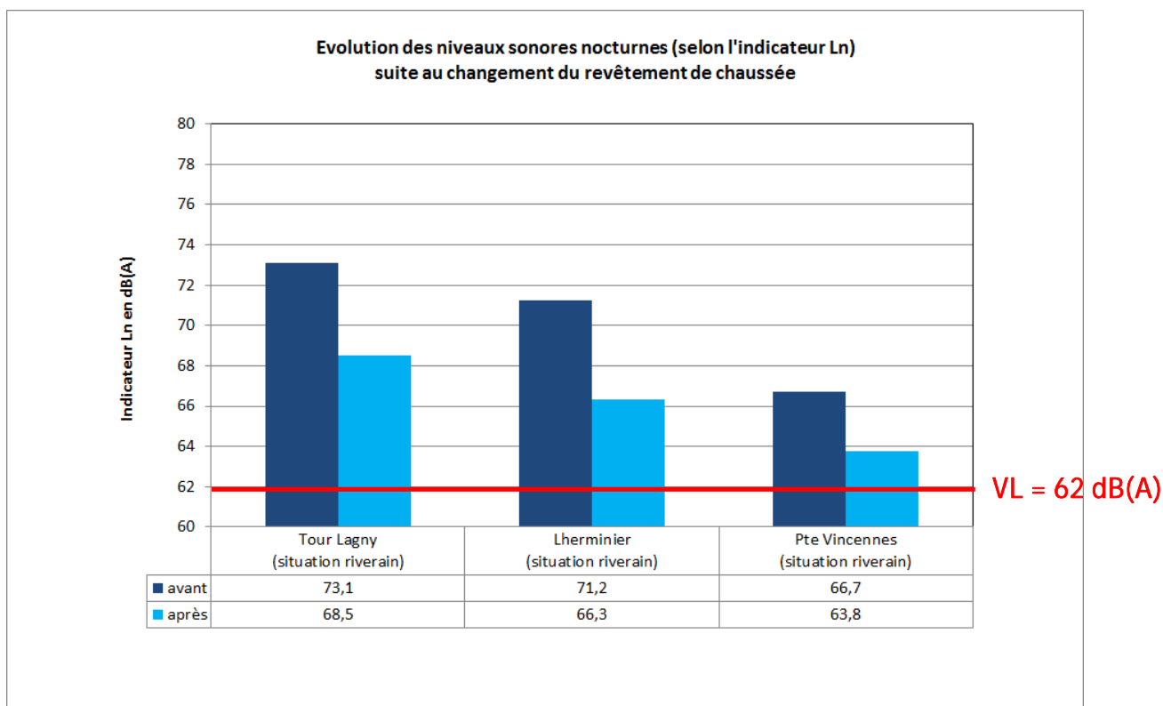
Figure 59 : Evolution de l'indicateur réglementaire Ln.
