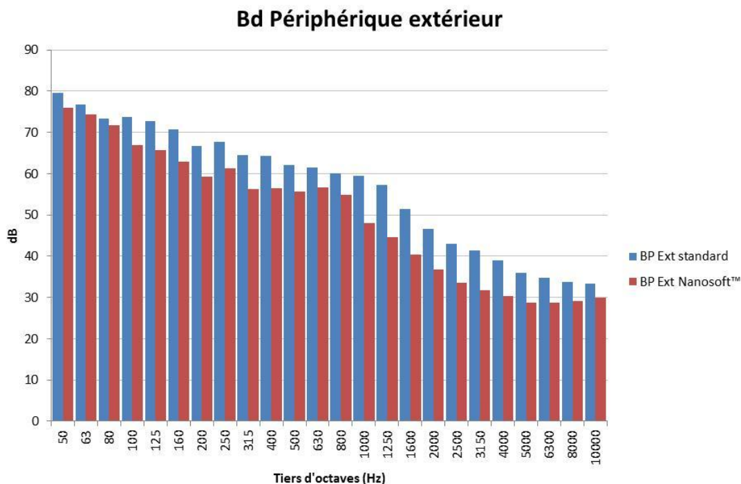
Figure 47 : Différence de spectre entre le bruit généré au passage sur l'ancien revêtement et le bruit généré au droit du nouveau revêtement Nanosoft® (au niveau du BPE).
