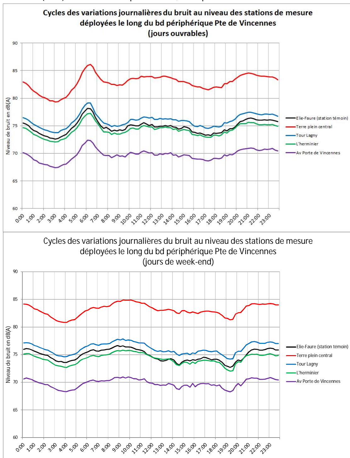
Figure 37 : Variations des niveaux de bruit au cours de la journée (en haut : jours ouvrables, en bas : jours de week-end).
