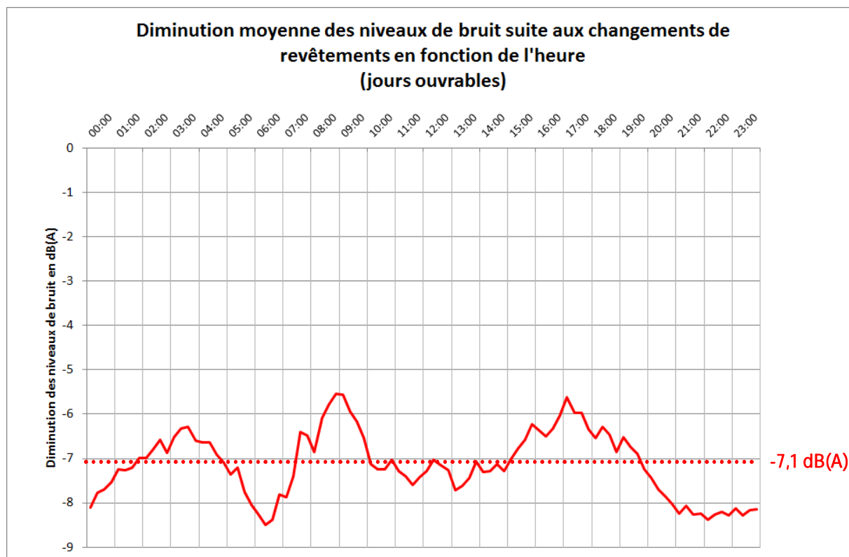
Figure 43 : Diminution des niveaux au cours d'un jour ouvrable type après la pose des revêtements en situation de proximité au trafic.
