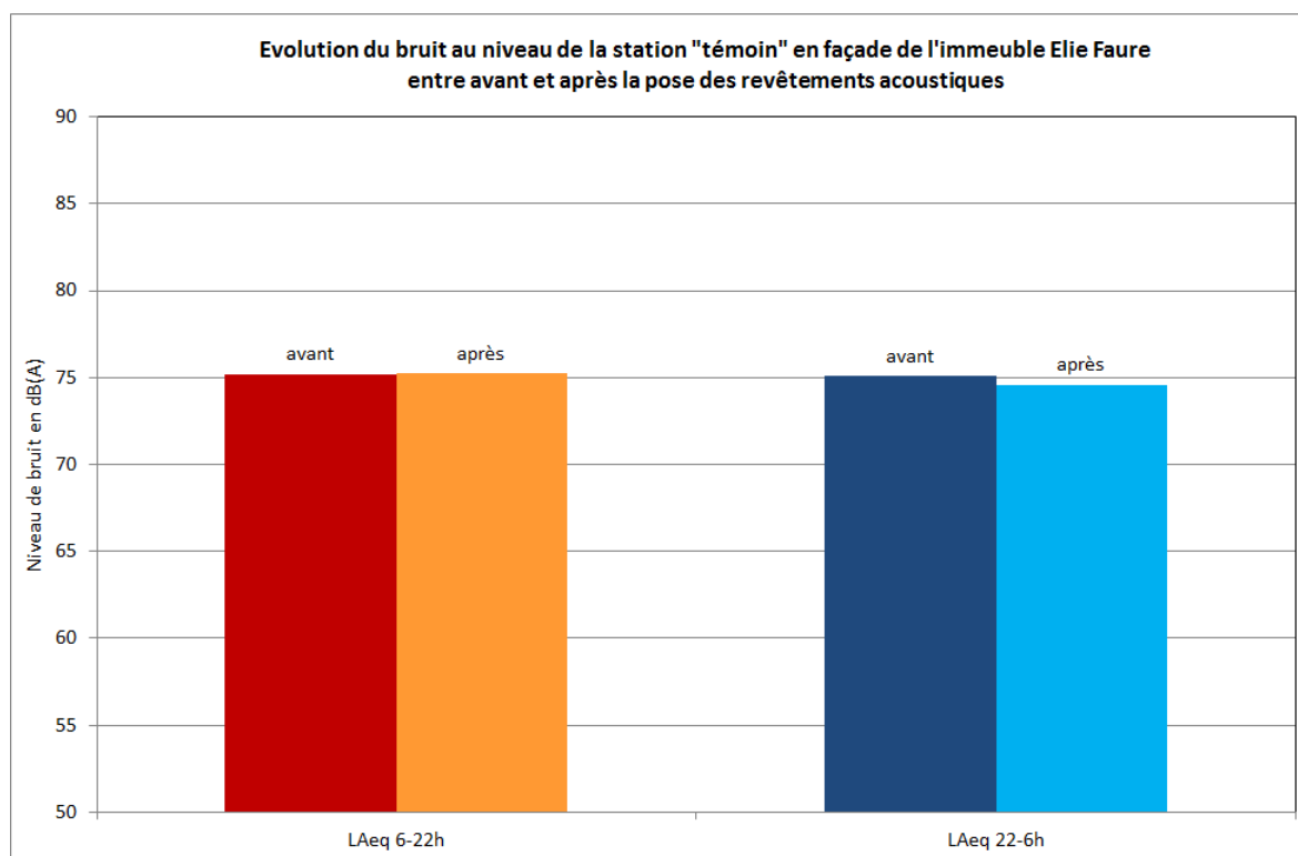
Figure 38 : Evolution des niveaux LAeq 6-22h et LAeq 22-6h entre les deux périodes sur la station « témoin » Elie Faure.
