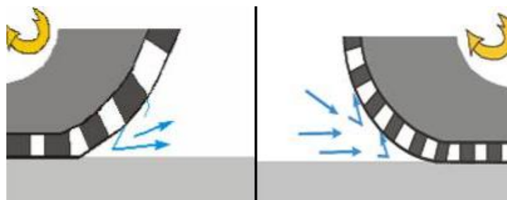
Figure 17 : Mécanisme de pompage d'air.
