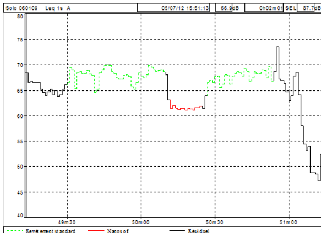
Figure 46 : Exemple d'évolution des niveaux sonores à l'intérieur de l'habitacle du véhicule Passage à 50 km/h sur le revêtement Nanosoft® BP extérieur : diminution de l'ordre de -7 dB(A).
