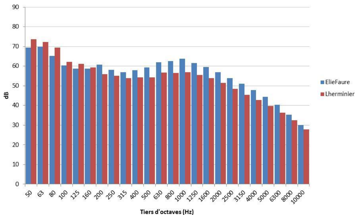
Figure 65 : Différence de spectre entre le bruit généré au droit de l'ancien revêtement (en situation riverain devant l'immeuble « témoin » Elie Faure) et le bruit généré au droit des nouveaux revêtements (en situation riverain devant l'immeuble l'Herminier).
