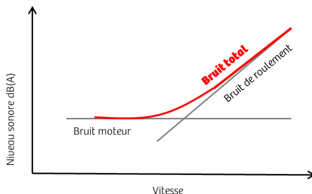
Figure 14 : Relation entre niveau sonore généré par un véhicule et sa vitesse.
