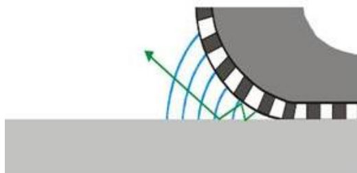
Figure 18 : Effet de corne ou « effet dièdre ».
