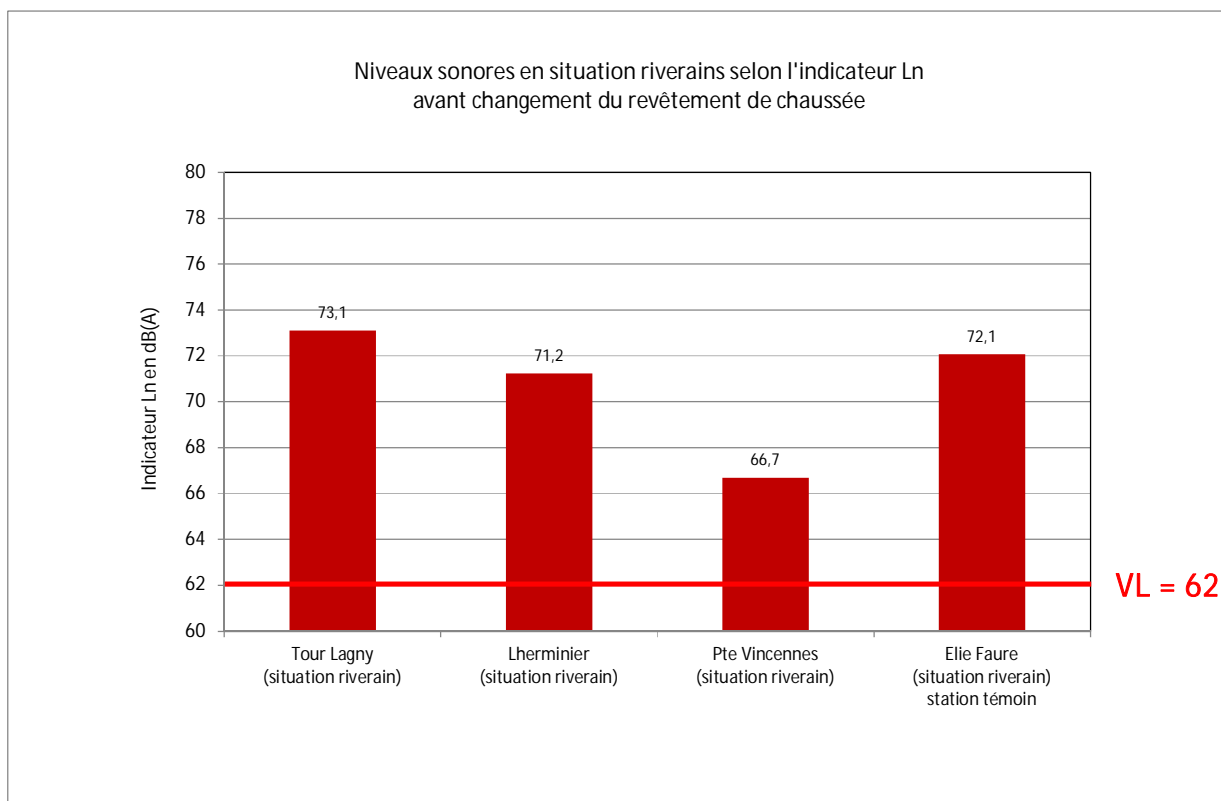
Figure 35 : Indicateurs Ln en situation « riverains ».
