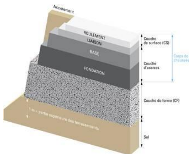
Figure 15 : Les différentes couches d'une chaussée.
