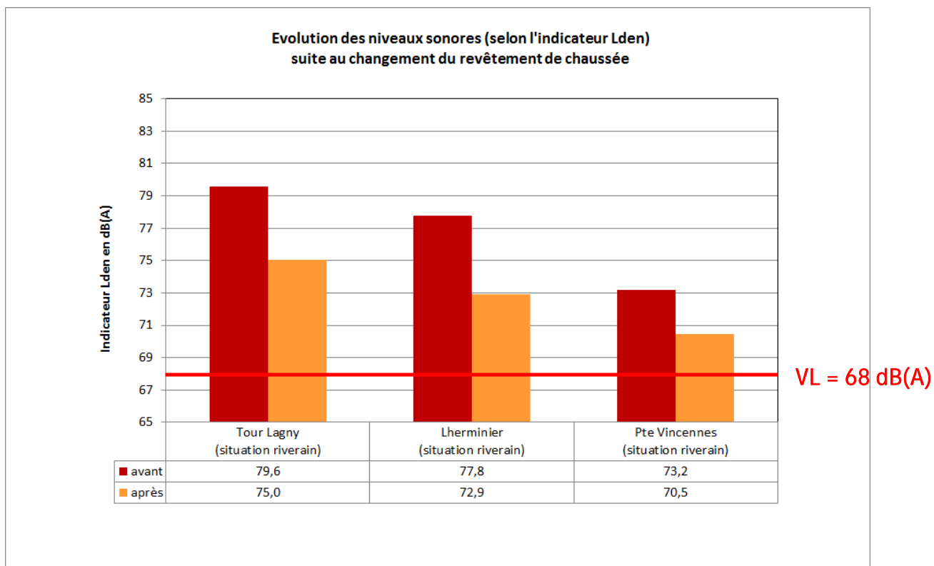
Figure 58 : Evolution de l'indicateur réglementaire Lden.
