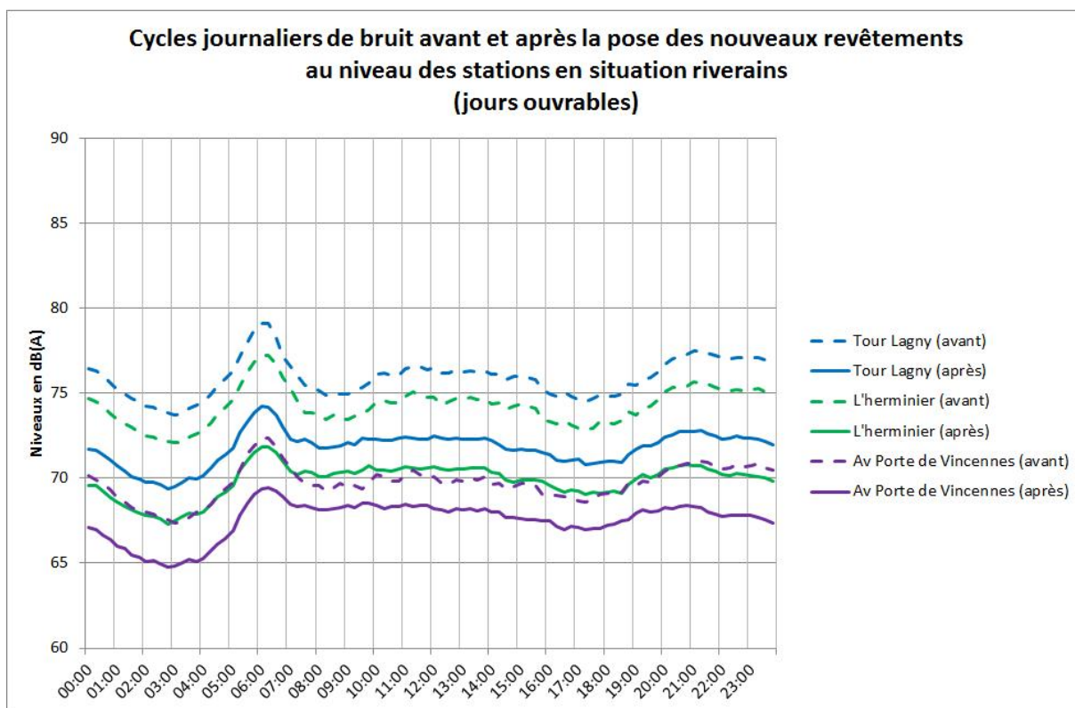
Figure 61 : Variation des niveaux au cours d'un jour ouvrable type avant et après la pose des revêtements en situation « riverains ».
