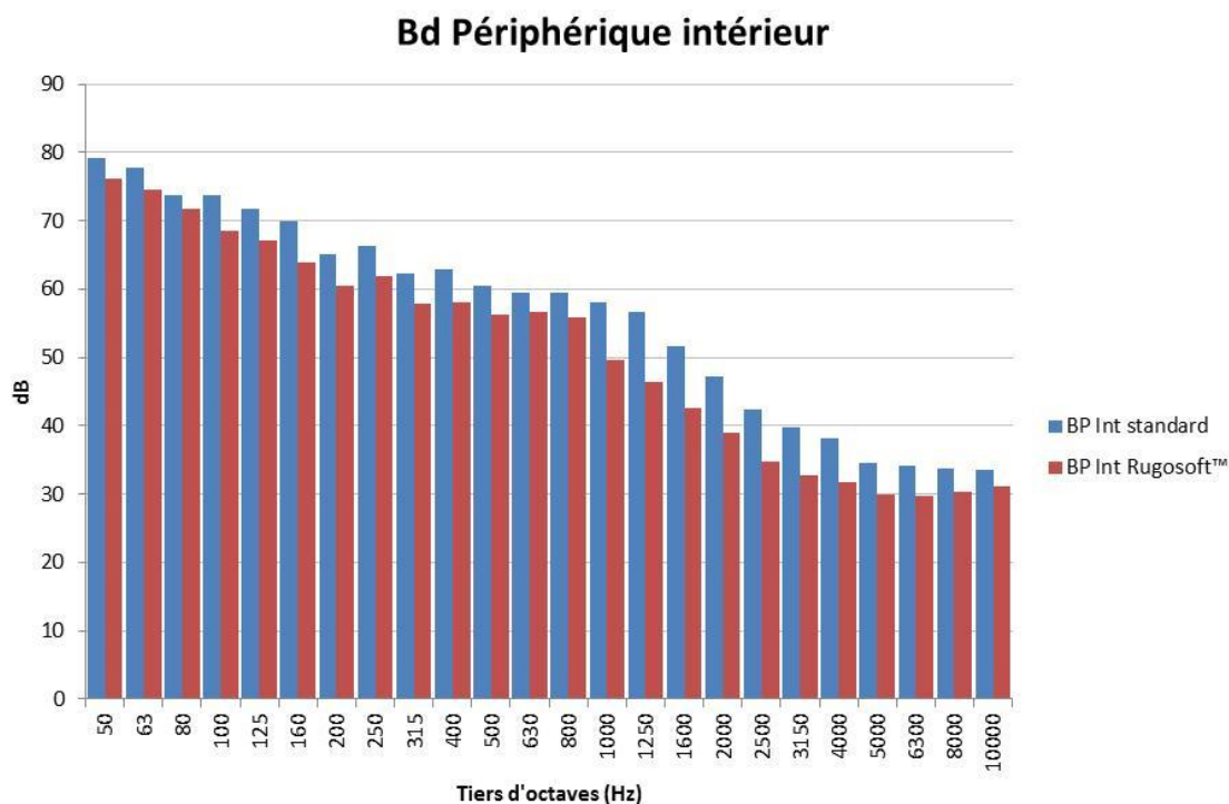
Figure 49 : Différence de spectre entre le bruit généré au passage sur l'ancien revêtement et le bruit généré au droit du nouveau revêtement Rugosoft® (au niveau du BPI).
