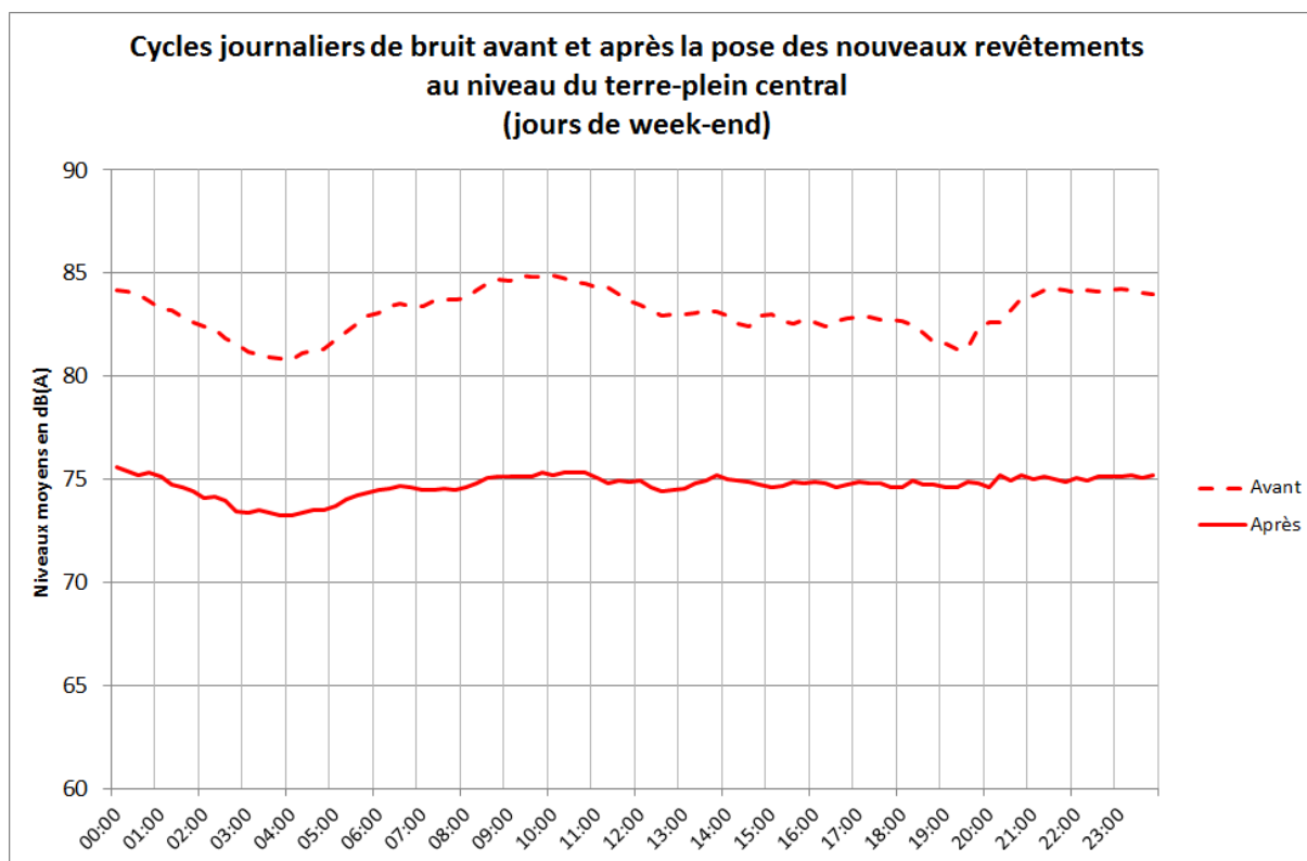
Figure 44 : Variation des niveaux au cours d'un jour week-end type avant et après la pose des revêtements en situation de proximité au trafic.
