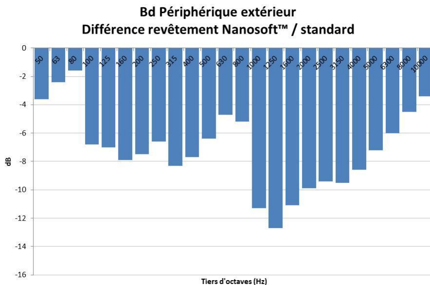
Figure 48 : Diminution des niveaux sonores au passage sur le revêtement Nanosoft® par rapport au revêtement standard.
