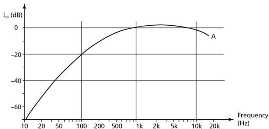
Figure 8 : Courbe de pondération fréquentielle A.
