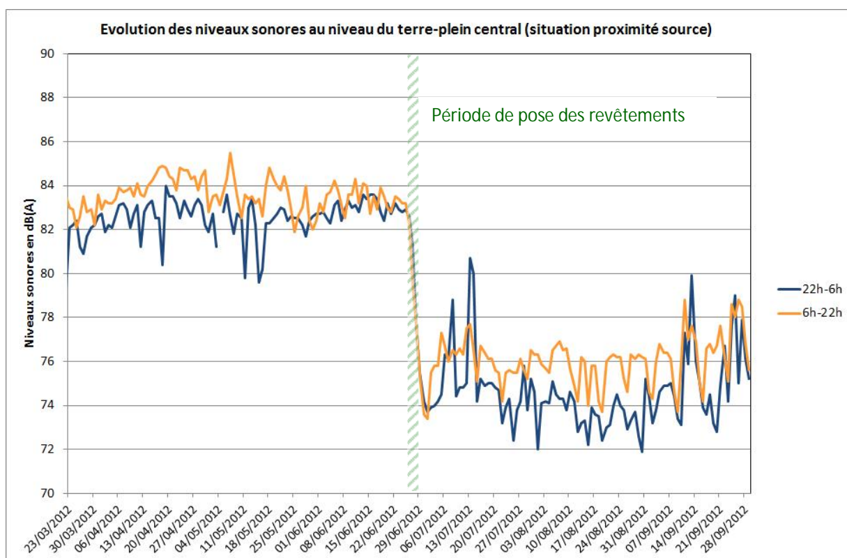
Figure 40 : Niveaux de bruit diurnes et nocturnes avant et après la pose des revêtements au niveau de la station de mesure située sur le terre-plein central.
