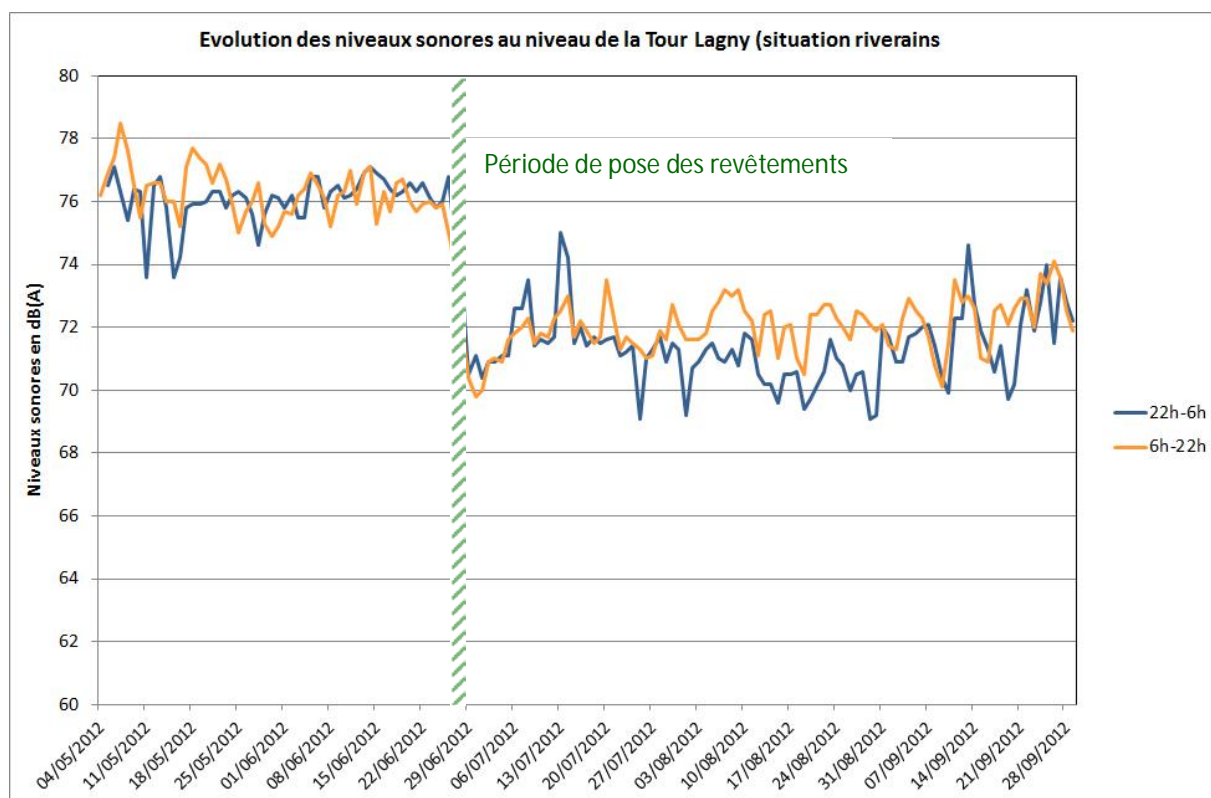
Figure 51 : Niveaux de bruit diurnes et nocturnes avant et après la pose des revêtements au niveau de la station de mesure située en façade de la Tour Lagny.
