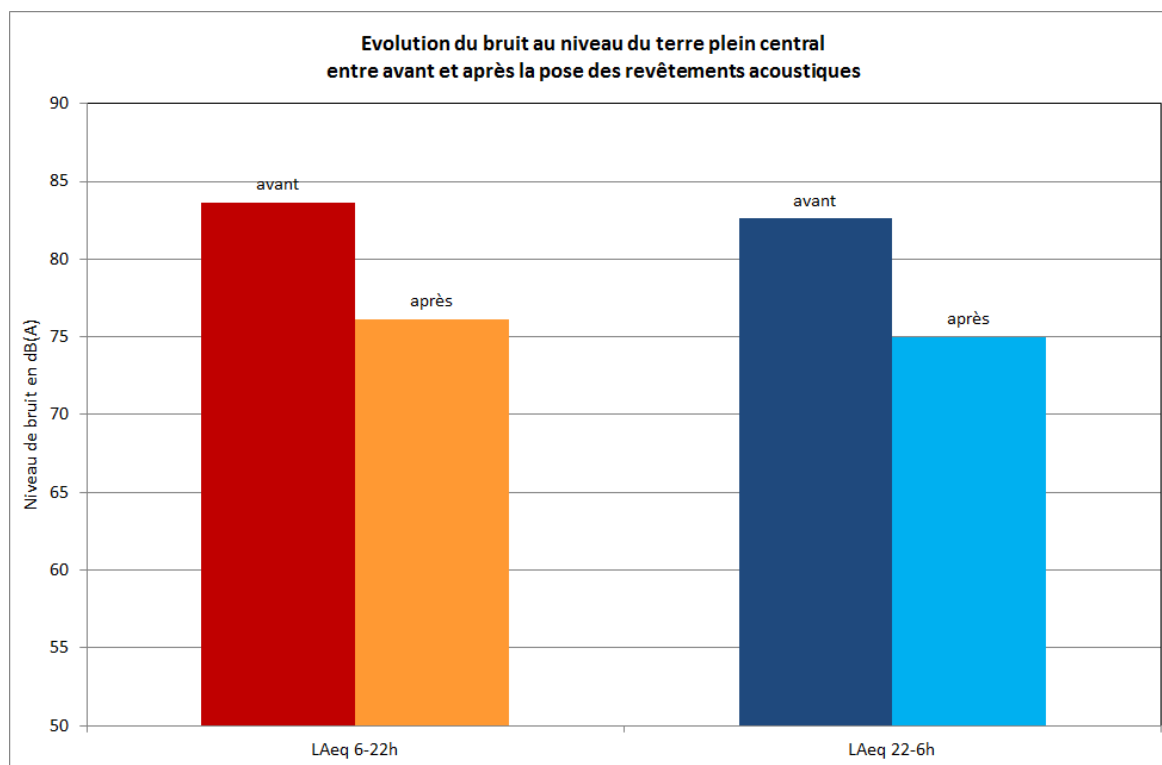
Figure 41 : Evolution des niveaux LAeq 6-22h et LAeq 22-6h entre les deux périodes sur la station située au niveau du terre-plein central.
