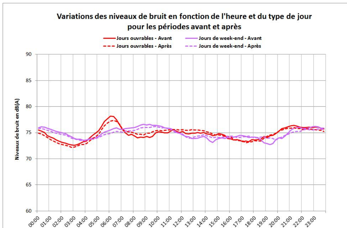
Figure 39 : Evolution des cycles moyens journaliers entre les deux périodes sur la station Elie Faure.
