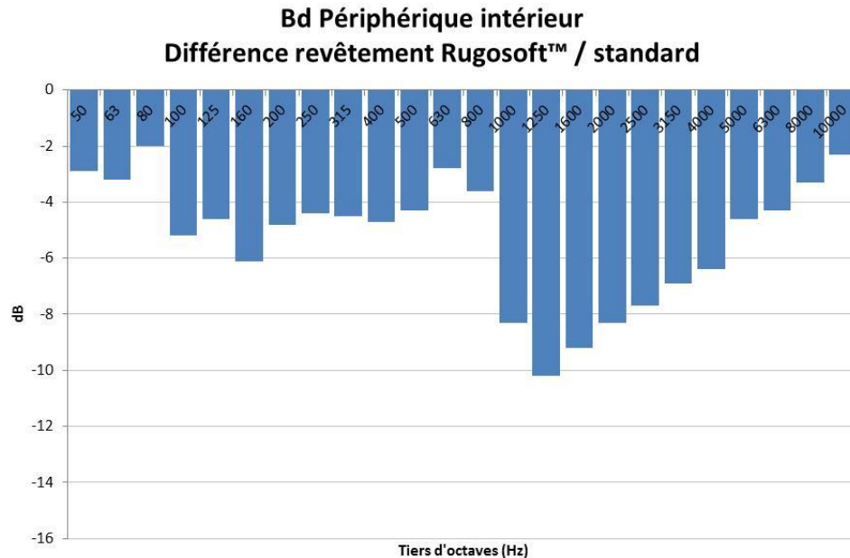
Figure 50 : Diminution des niveaux sonores au passage sur le revêtement Rugosoft® par rapport au revêtement standard.
