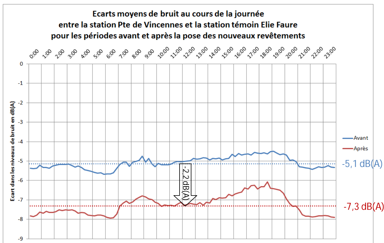
Figure 54 : Ecarts moyens de bruit au cours de la journée entre les stations « riverains » du secteur d'expérimentation et la station témoin.
