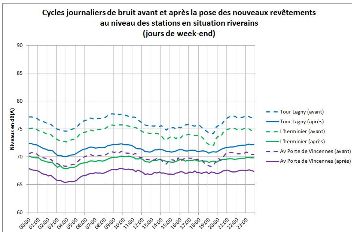
Figure 63 : Variation des niveaux au cours d'un jour de week-end type avant et après la pose des revêtements en situation « riverains ».
