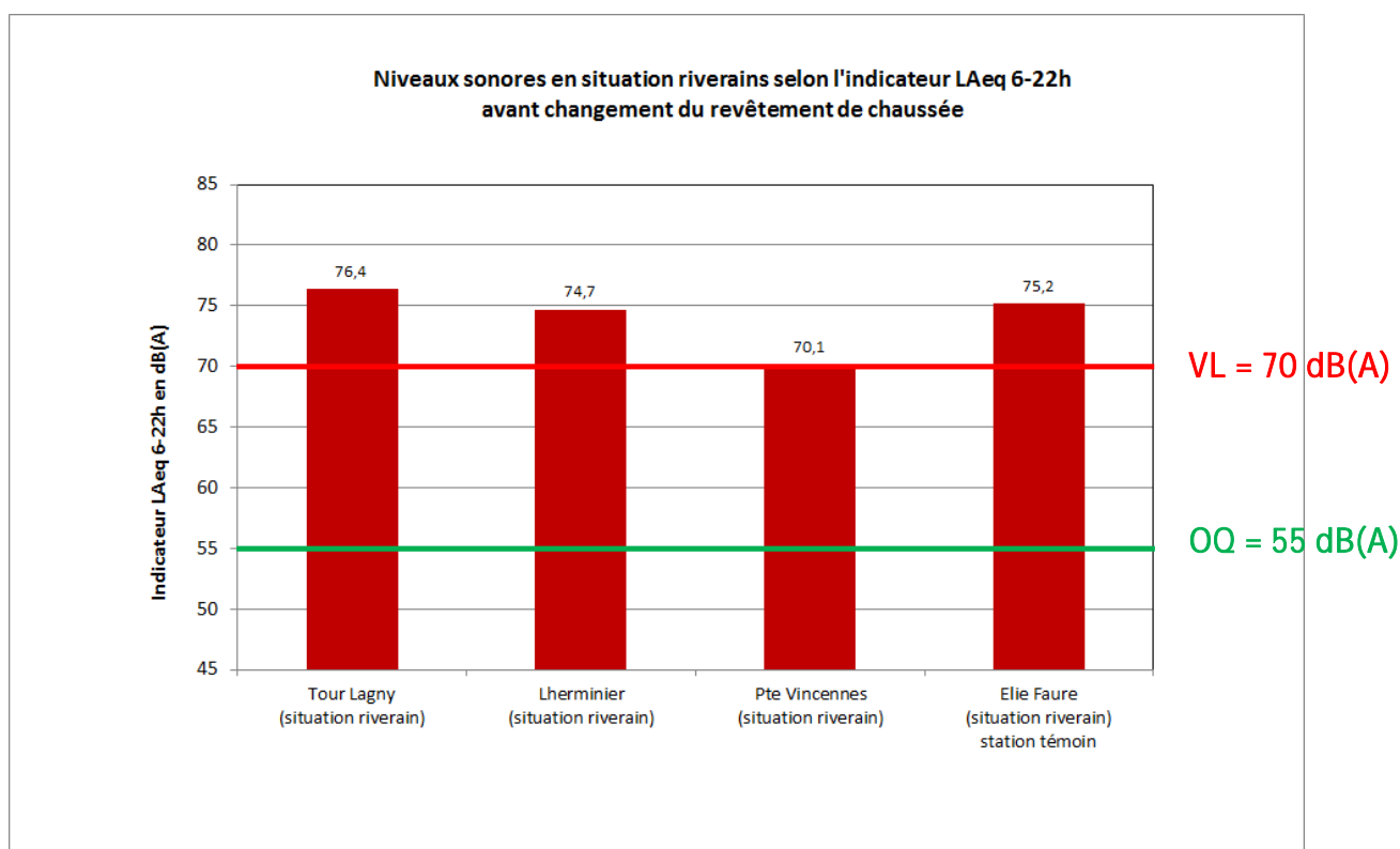
Figure 33 : Indicateurs LAeq 6-22h en situation « riverains ».
