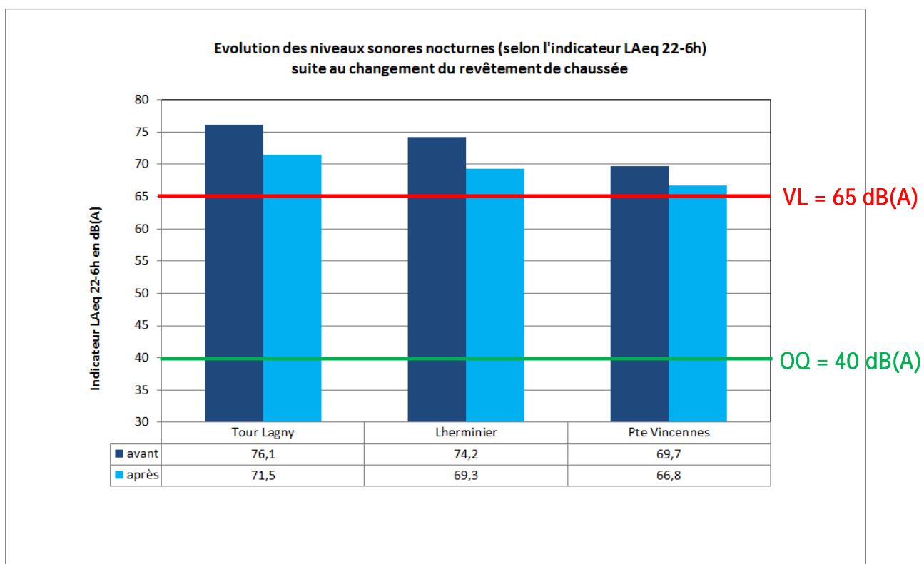
Figure 57 : Evolution de l'indicateur réglementaire LAeq 22-6h.
