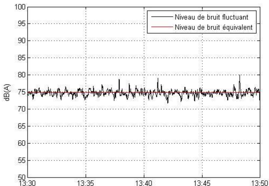
Figure 5 : Evolution temporelle du niveau de bruit et niveau continu équivalent.
