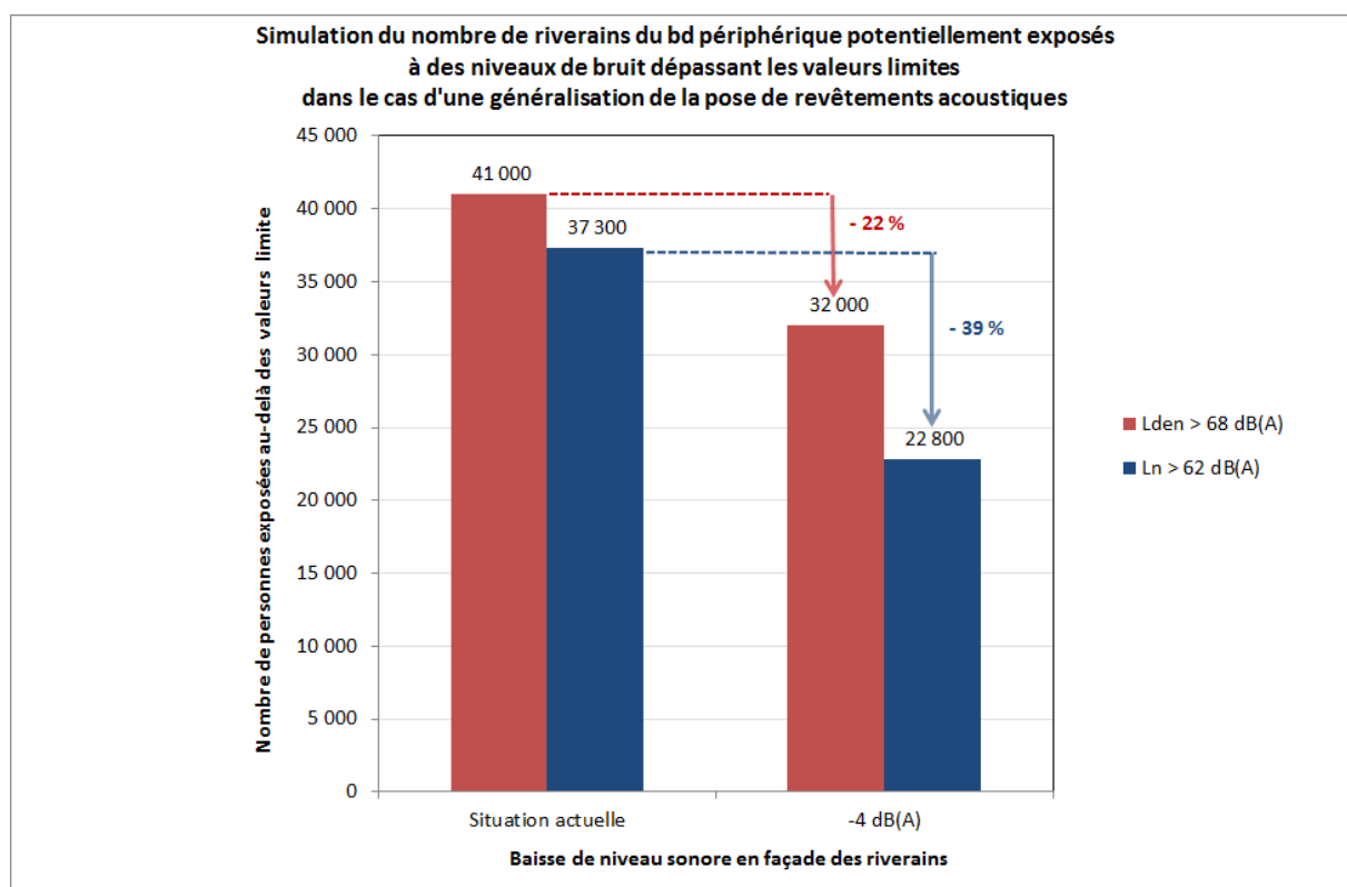
Figure 60 : Simulation de l'impact en termes de riverains du bd périphérique exposés à des niveaux excédant les valeurs limites en cas de généralisation des revêtements acoustiques.
