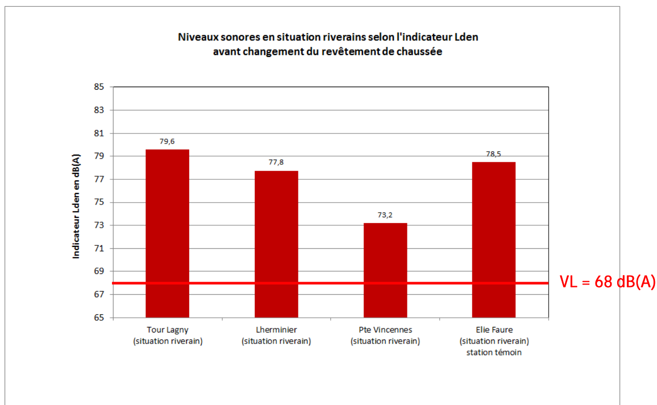
Figure 36 : Indicateurs Ln en situation « riverains ».
