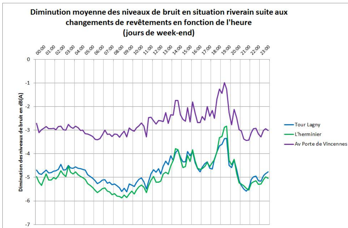
Figure 64 : Diminution des niveaux au cours d'un jour de week-end type après la pose des revêtements en situation « riverains ».
