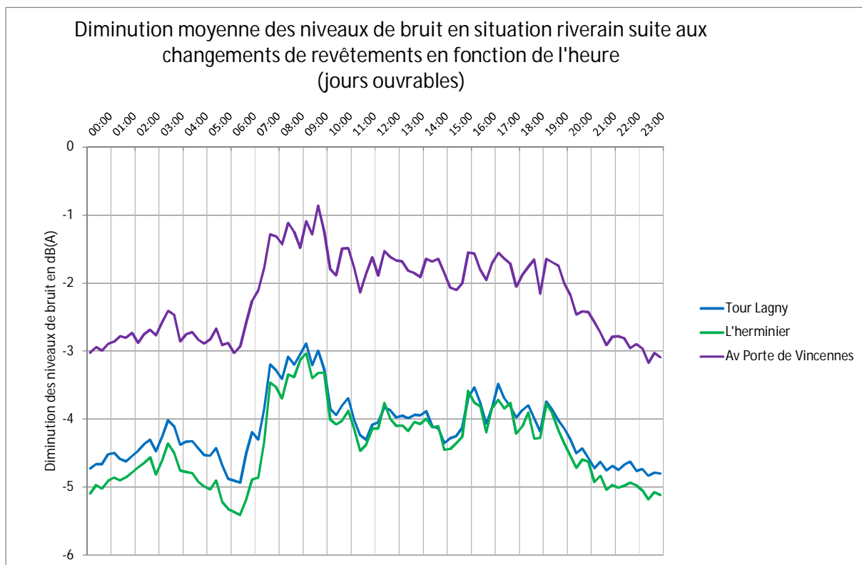
Figure 62 : Diminution des niveaux au cours d'un jour ouvrable type après la pose des revêtements en situation « riverains ».
