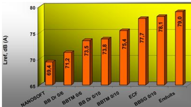
Figure 19 : Diagramme extrait de la base de données du LRPC (valeurs moyennes des mesures L max réalisées en véhicules isolés (VI), à 90 km/h, par famille de revêtements) ; source : Notice technique Nanosoft®, Colas (2010).
