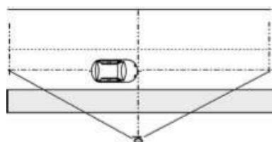
Figure 20 : Procédure de mesure "au passage".
