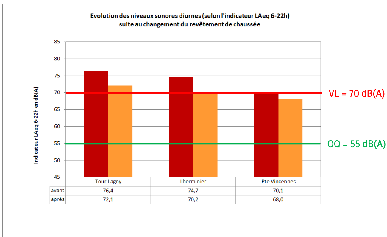
Figure 56 : Evolution de l'indicateur réglementaire LAeq 6-22h.
