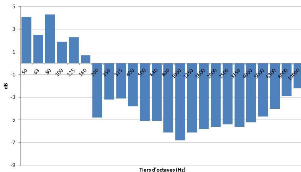
Figure 66 : Diminution des niveaux sonores par bande de tiers d'octave entre la situation riverains côté nanosoft® BPE devant l'immeuble l'Herminier et la situation riverains côté BPE devant l'immeuble « témoin » Elie Faure.
